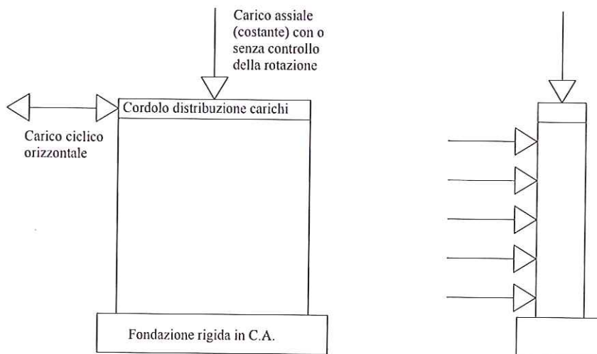
Figura 10-5: Prove tipo 5 (opzionale) - Prototipi per prove sperimentali con applicazione combinata delle azioni nel piano e fuori piano. Si noti che nella figura i cordoli e gli elementi di fondazione hanno il solo scopo di consentire l'applicazione del carico in fase di prova e non sono parte integrante dell'elemento strutturale considerato nello studio
