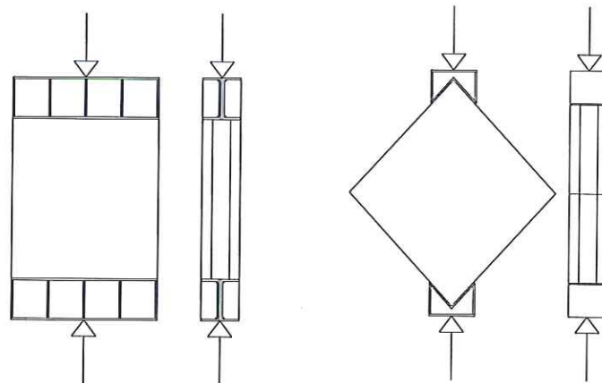
Figura 10-1: Prove tipo 1 - Prototipi di dimensioni ridotte (indicativamente 1.0 m x 1.0 m), determinazione del modulo elastico
