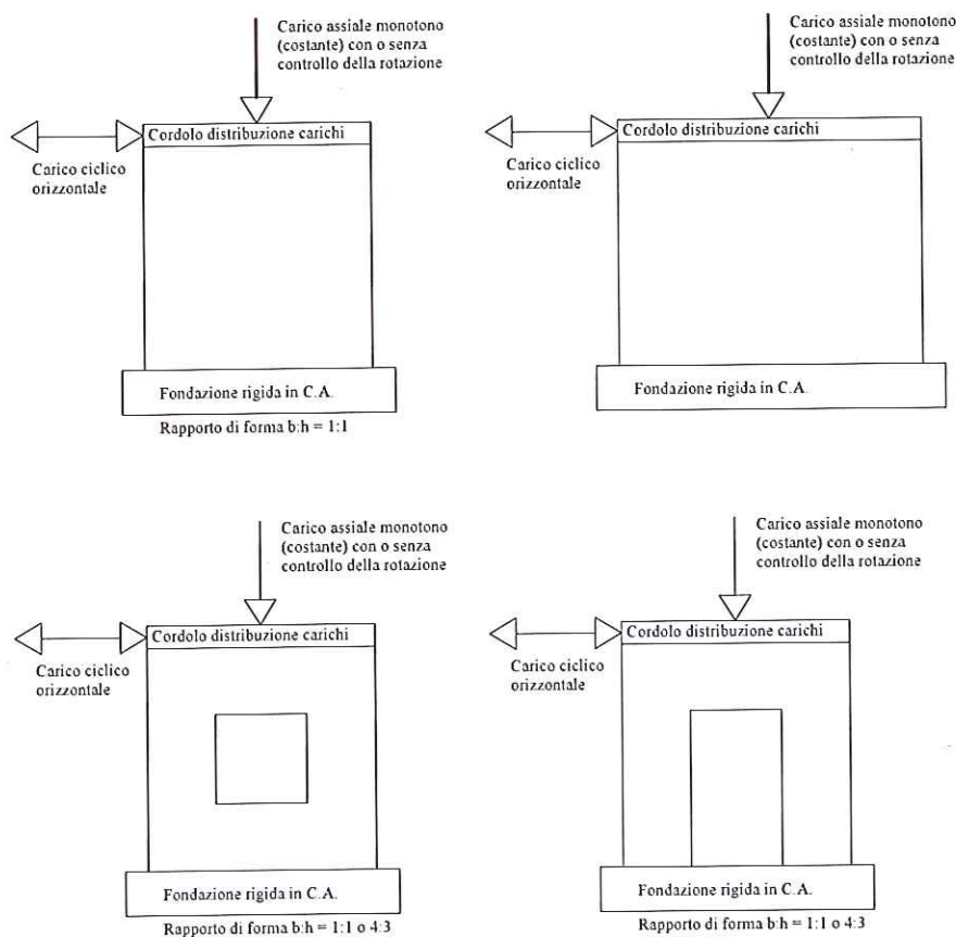
Figura 10-2: Prove tipo 2 - Prototipi di pannelli in scala reale (indicativamente h =altezza interpiano tipo, b \geq 1.0 m), valutazione del carico di collasso per instabilità locale e globale del pannello
