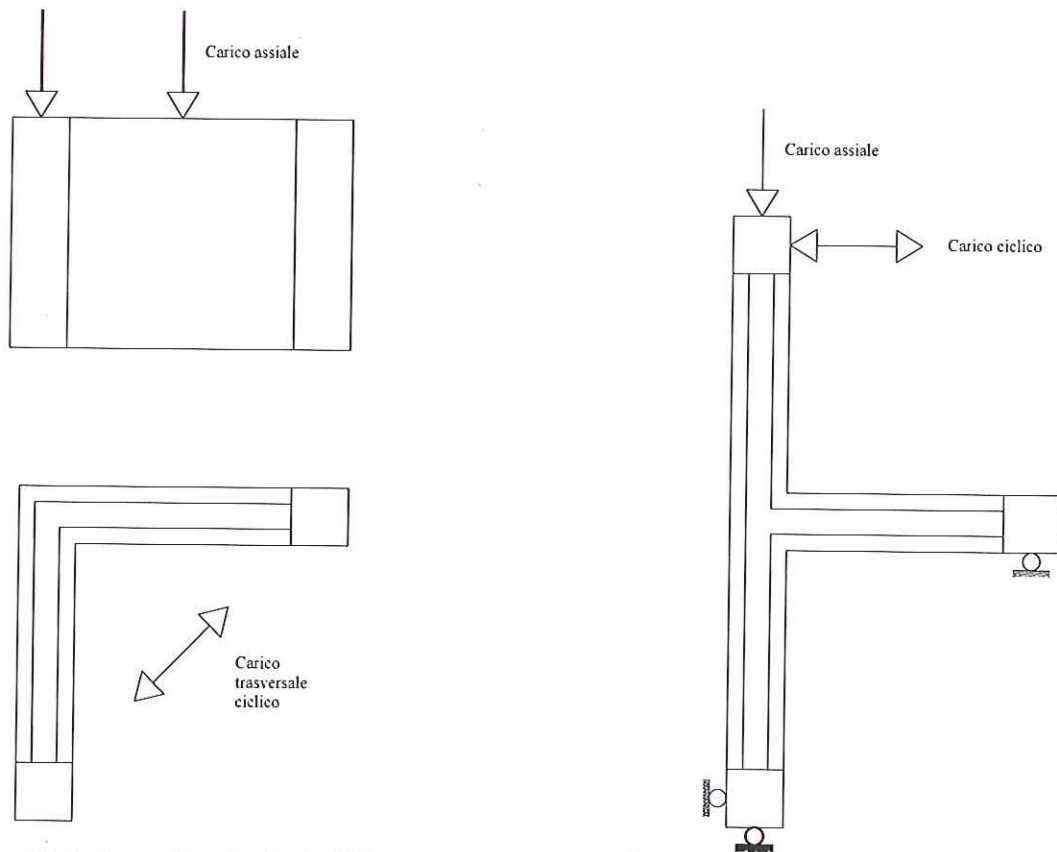
Figura 10-4: Prove tipo 4 - Prototipi per prove sperimentali sulle connessioni ad L e T.
