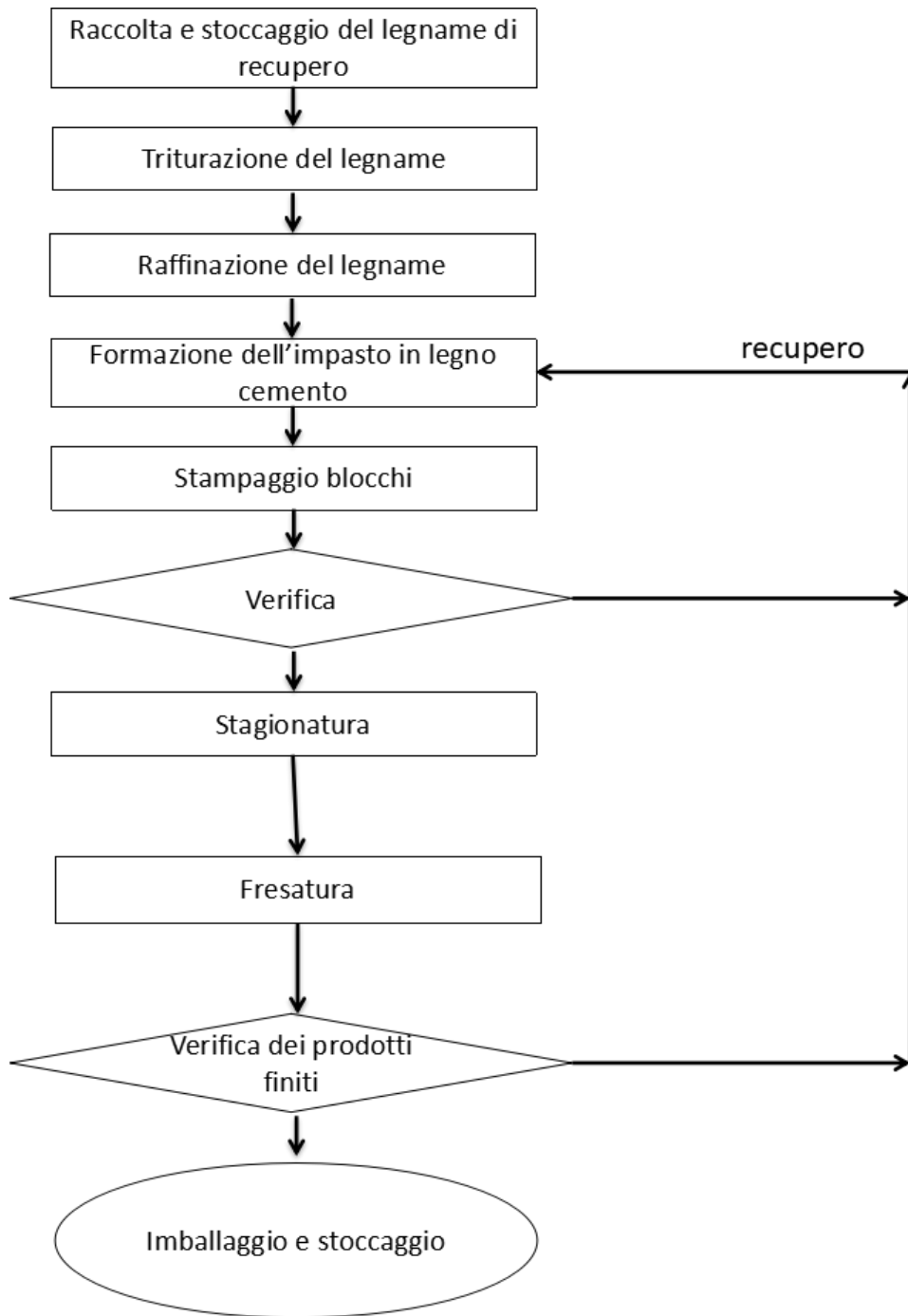
Figura 2: Il processo produttivo per la realizzazione degli elementi per barriere acustiche in legno cemento ISOTEX
