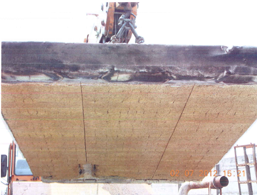
Foto 4. Lato esposto al fuoco del solaio dopo la prova
